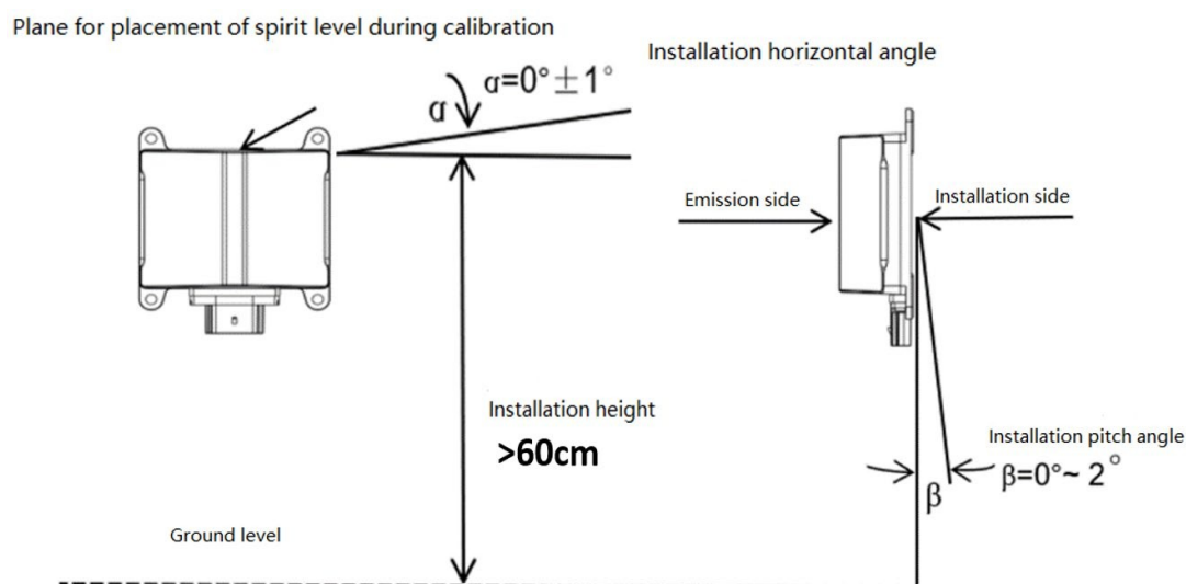
Figure 2-3 Diagramme de déviation de l'installation du radar
